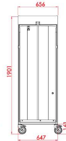
Logist'ALLI F600 18G Motorisée
