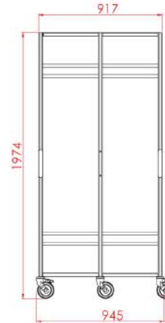
Stock'ALI 2x400 21G
