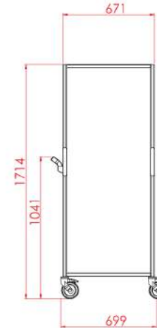
Stock'Ali F600 18G
