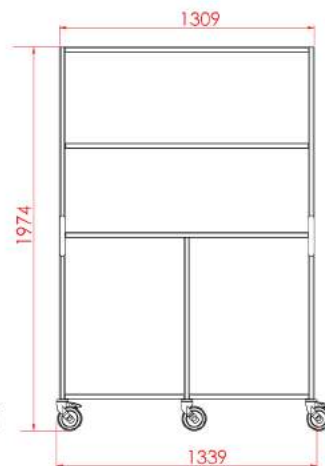
Stock'Ali F1200 Mixte ou F1200
