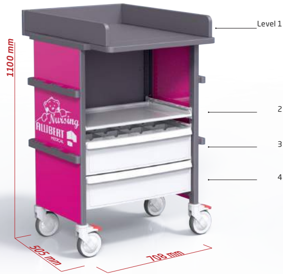
Baby changing cart V2
