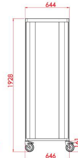
Mod'Alli F600 21G
